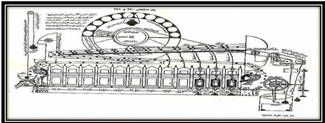
مخطط الساعة الميكانيكية متعددة الوظائف التي بناها رضوان الساعاتي في المسجد الأموي بدمشق
